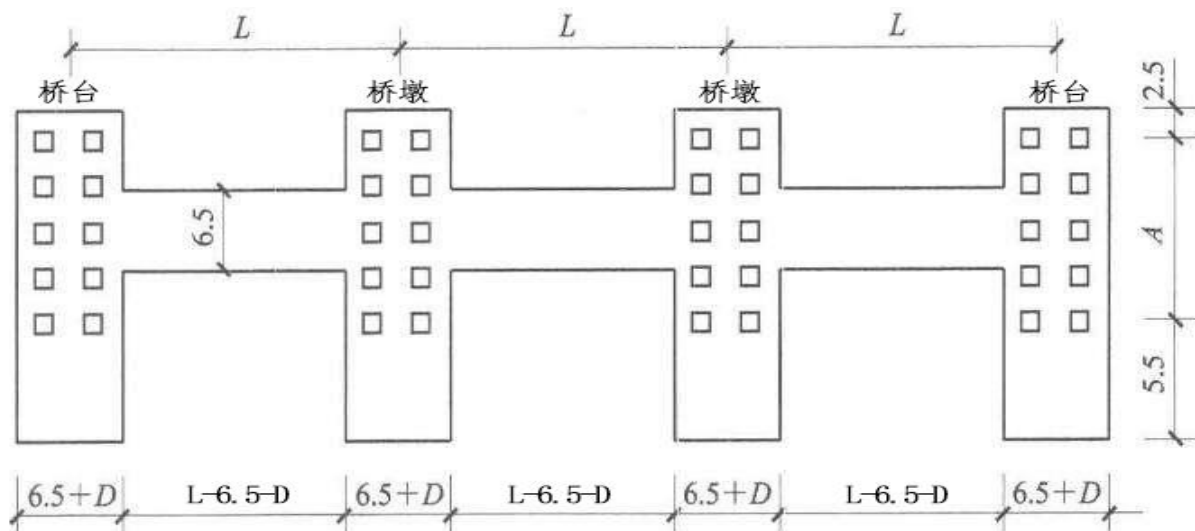
工作平台面积计算示意图
